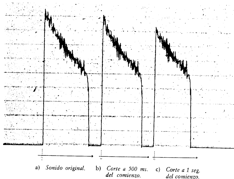
FIG. 6 (parágrafo VII.3).—Batigramas de corte para un la, del piano. a) La pendiente media de la dinámica descendente es constante. b) y c) Los sonidos cortados hacen oír sensiblemente el mismo ataque que el sonido original.
