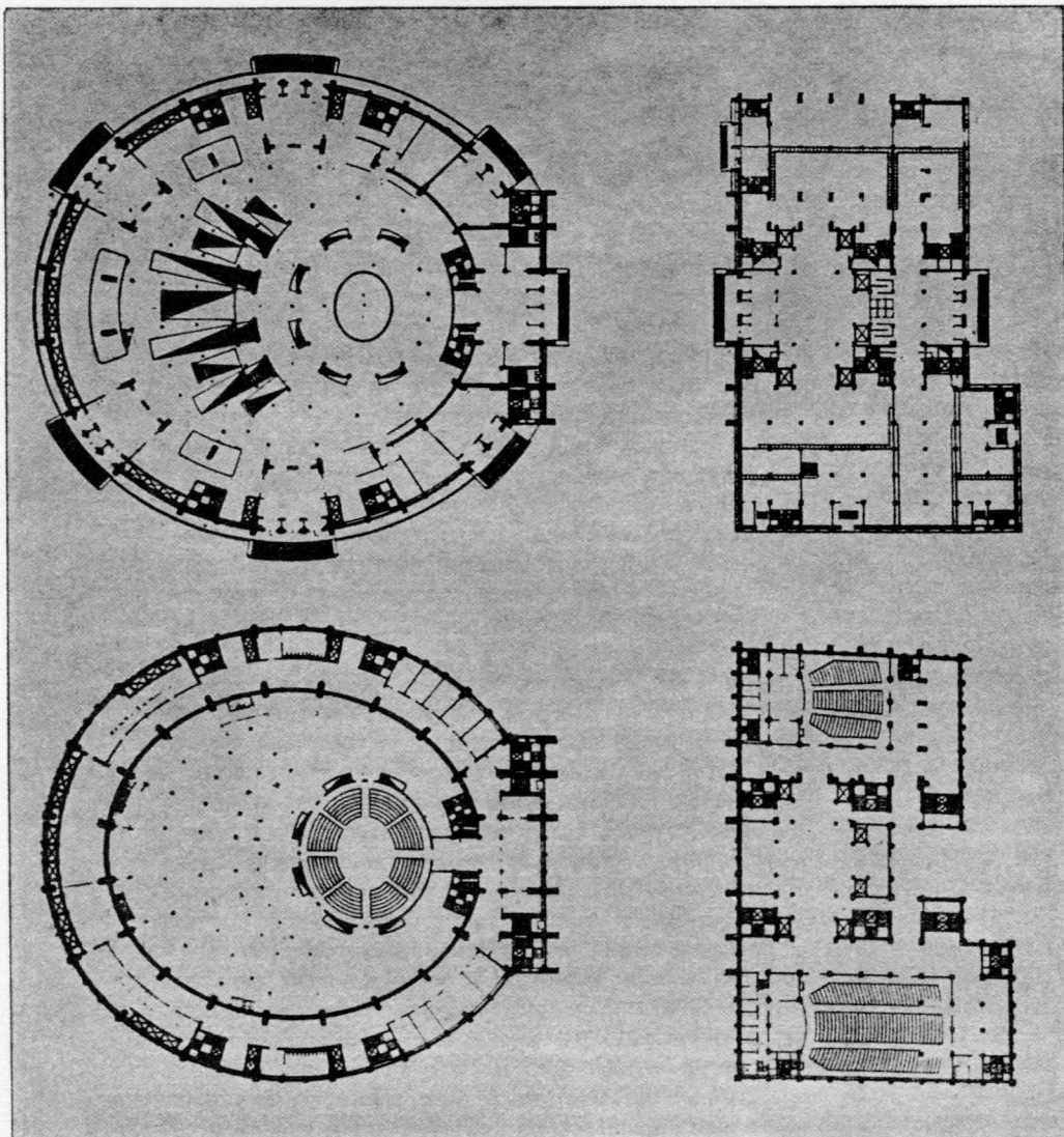
L., A. UND V. WESNIN. ENTWURF DES „PALAIS DER ARBEIT“ IN MOSKAU. 1923
