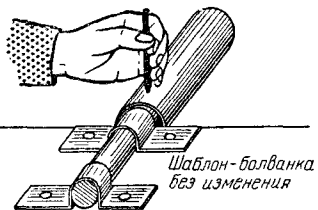
КЛЕПКА ТРУБКИ установочная фаза № 4
