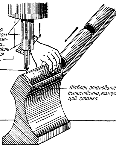
КЛЕПКА (ПРЕССОВКА) ТРУБКИ установочная фаза № 7
