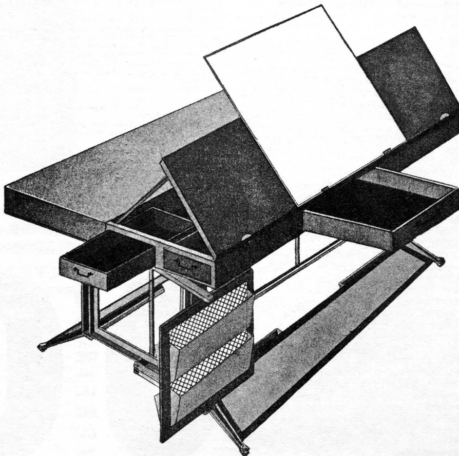
СТОЛ предназначен для письменной работы, черчения и обеда. В нижнюю часть стола могут убираться 4 складные стула, а также из нижней части (подставки) выдвигаются с обеих сторон конверты для журналов, газет и бумаг. Крышка одной половины стола поднимается вместе с боковыми сторонами и, занимая вертикальное положение, открывает стол для обеда, на котором имеется передвижная в прорезах дорожка (скатерть).
