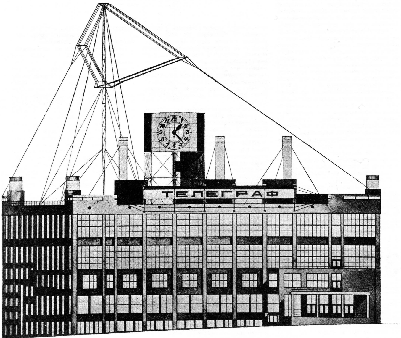
Фасад по Тверской улице
