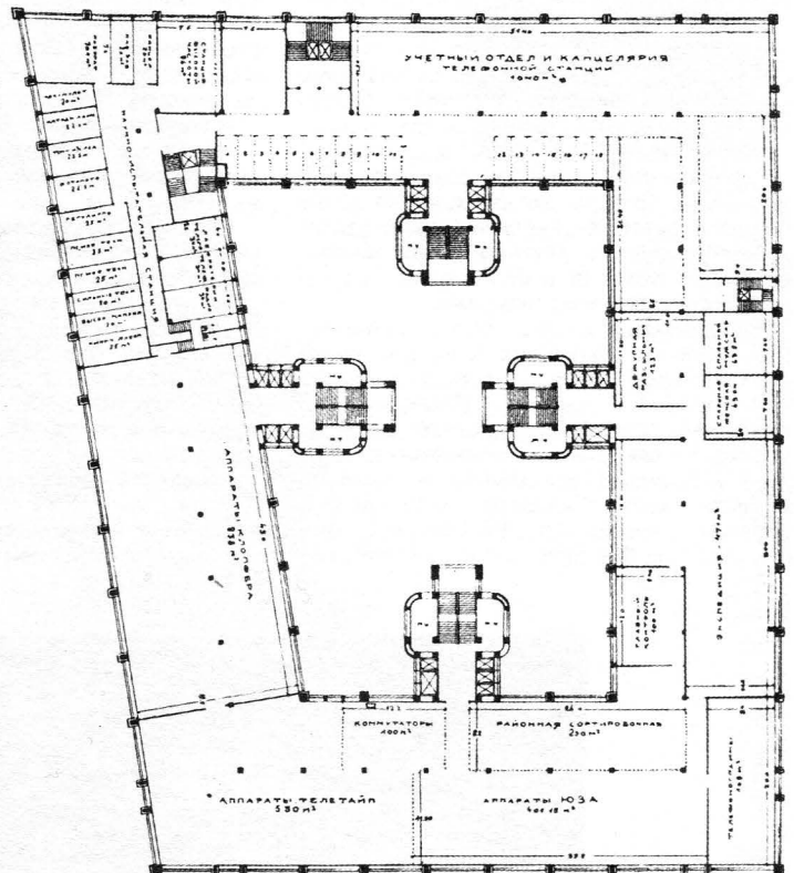
План 3-го этажа
