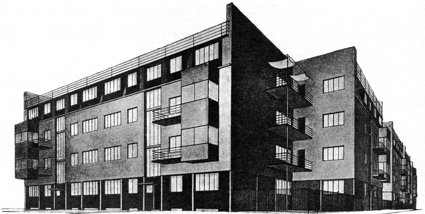
А. Буров и М. Парусников. Москва. Конкурсный проект рабочих домов для Иванова-Вознесенска. A. Burov und M. Parusnikoff. Moskau. Entwurf für Arbeiterhäuser in Iwanowo-Wonessensk. Типовой блочно-серийный дом, составленный из 12 блоков по две 3-комнатные квартиры на 6 человек каждая (по 9.18 м. на человека), по заданию 3 этажа, 4 мансардный с использованием крыши. Комбинация блоков может переставляться любым образом в зависимости от каждого частного случая задания, конфигурации и ориентировки генерального плана. Новый прием разрешения фасада жилого дома является результатом стандартизации всех элементов и блочно-серийного типа здания
