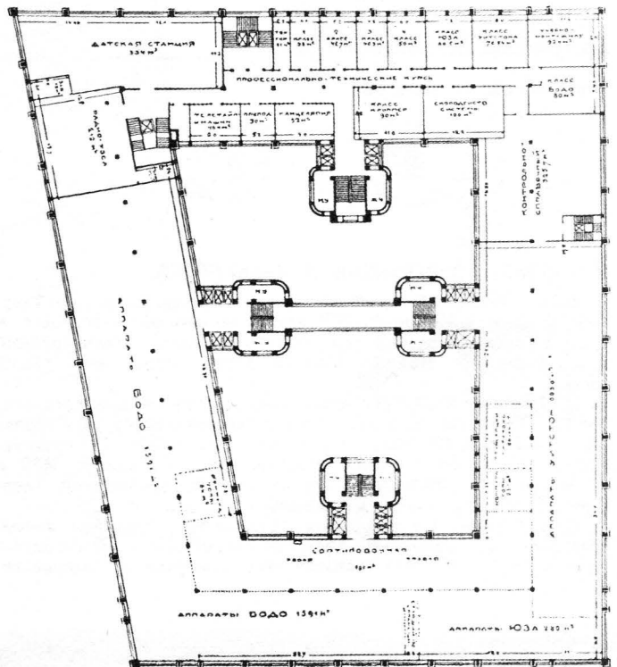
План 4-го этажа.
