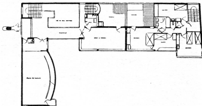
2-й этаж
