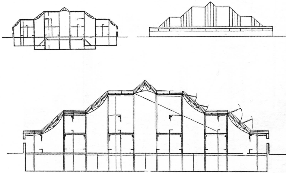
М. Я. Гинзбург при участии В. Н. Владимиров. Москва. Конкурсный проект крытого рынка. М. Ginsburg bei Teilnahme W. Wladimiroff. Moskau. Entwurf einer Markthalle
