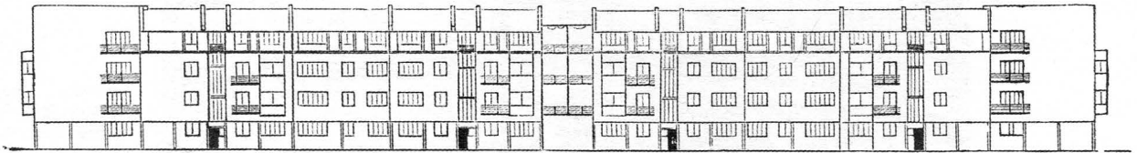
А. Буров и М. Парусников. Москва. Конкурсный проект рабочих домов для Иванова-Вознесенска. A. Burov und M. Parusnikoff. Moskau. Entwurf für Arbeiterhäuser in Iwanowo-Wonessensk. Типовой блочно-серийный дом, составленный из 12 блоков по две 3-комнатные квартиры на 6 человек каждая (по 9.18 м. на человека), по заданию 3 этажа, 4 мансардный с использованием крыши. Комбинация блоков может переставляться любым образом в зависимости от каждого частного случая задания, конфигурации и ориентировки генерального плана. Новый прием разрешения фасада жилого дома является результатом стандартизации всех элементов и блочно-серийного типа здания
