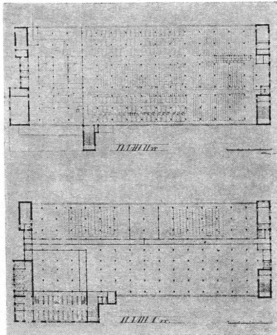
Планы
