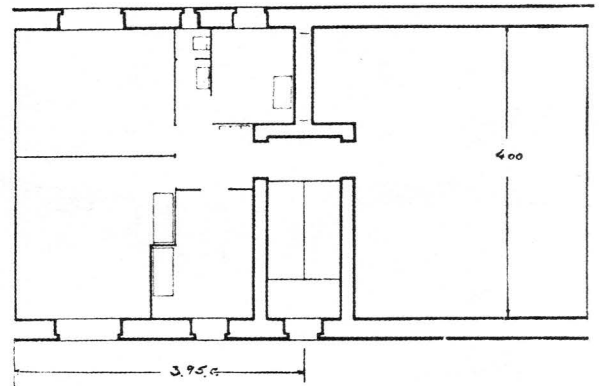
Типовая ячейка со сквозным проветриванием
