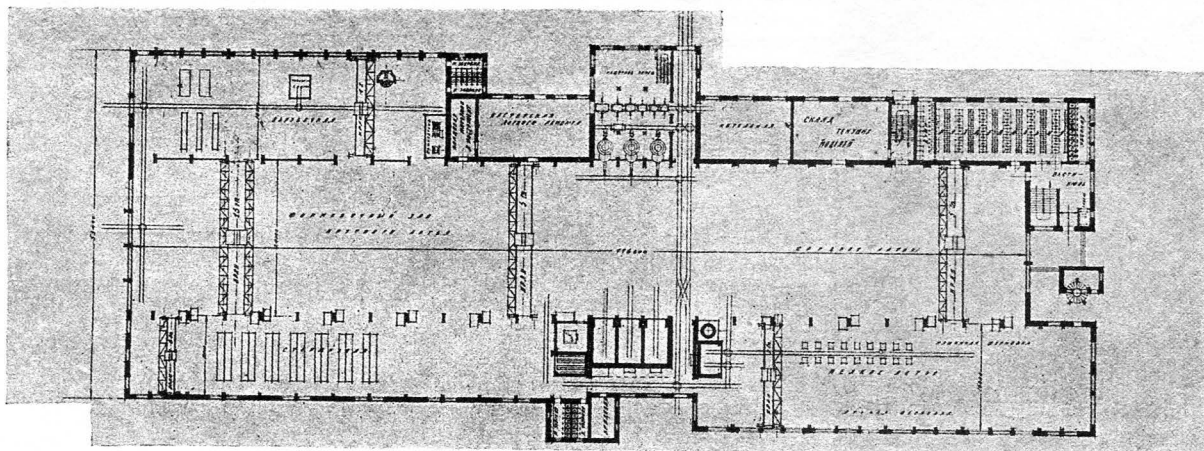
План
