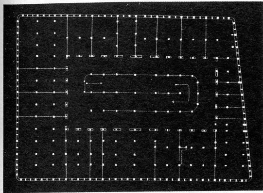
План нижнего подвала
