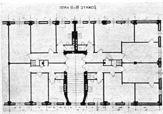
Типовая ячейка без сквозного проветривания
