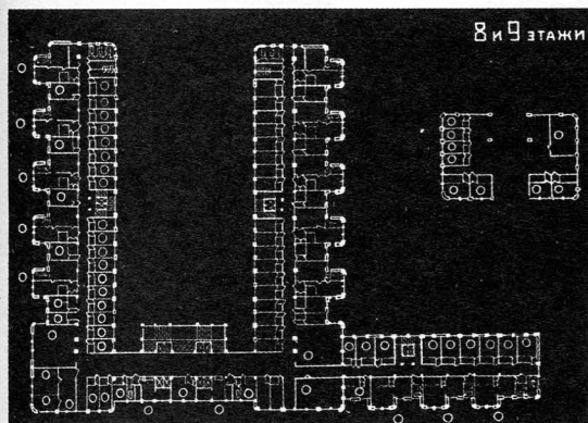
План 8 и 9 этажей
