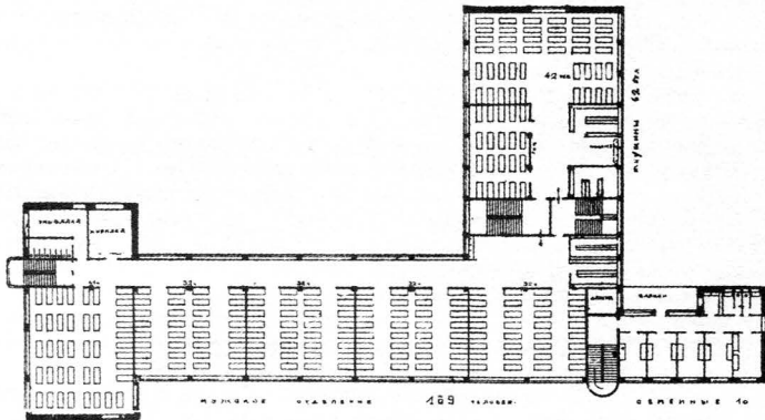
План верхних этажей
