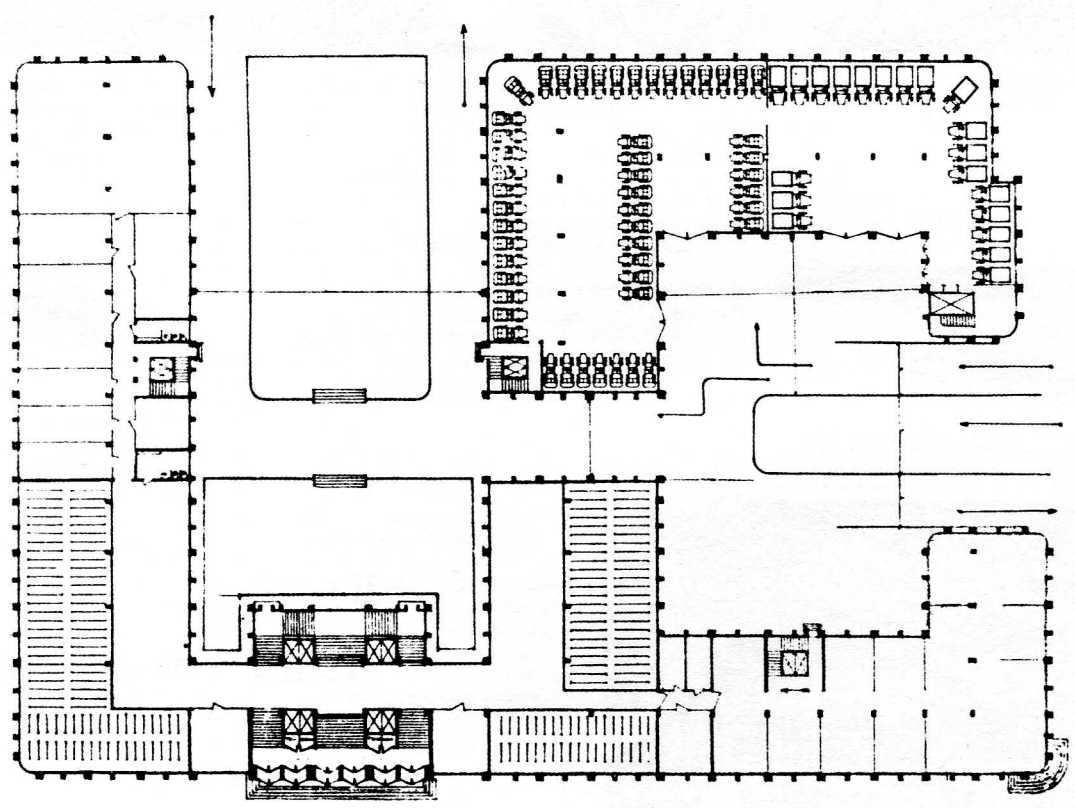
План полуподвала
