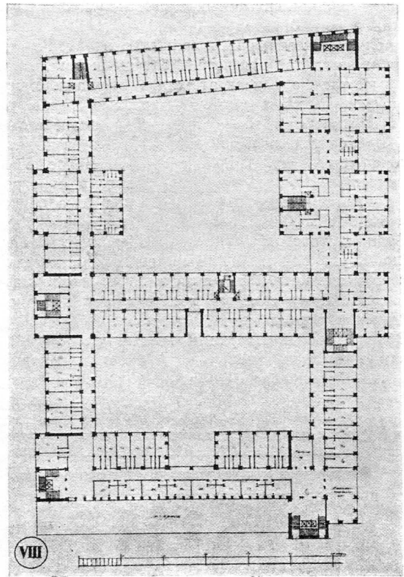
План 8-го этажа
