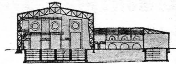
Разрез
