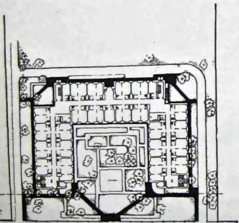
А. С. ФУФАЕВ. ПРОЕКТ РАБОЧИХ ДОМОВ
