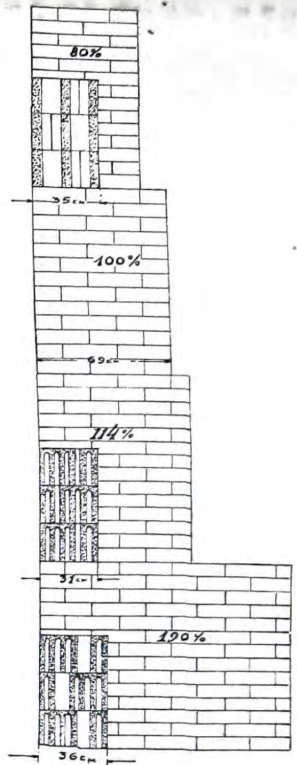
ПОКАЗАТЕЛЬ СООТНОШЕНИЯ ТОЛЩИНЫ СТЕН И ИХ ТЕПЛООВОГО КОЭФФИЦИЕНТА
