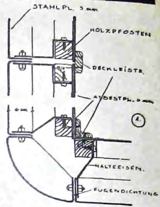
АНГЛИЙСКАЯ СИСТЕМА СТАЛЬНЫХ ДОМОВ
