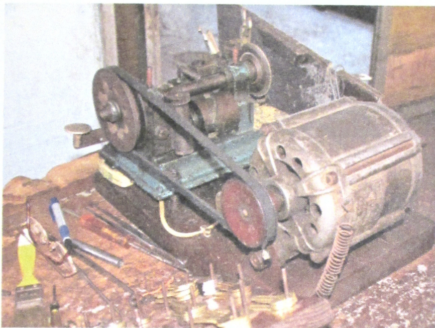
Moteur de machine à laver Aurika utilisé comme outil pour dupliquer des clés.
