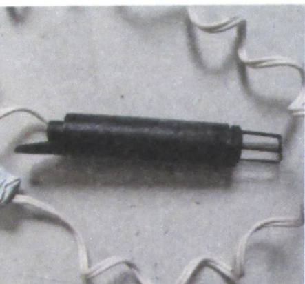
Allume-gaz qui fonctionne sur le principe du court-circuit électrique.
