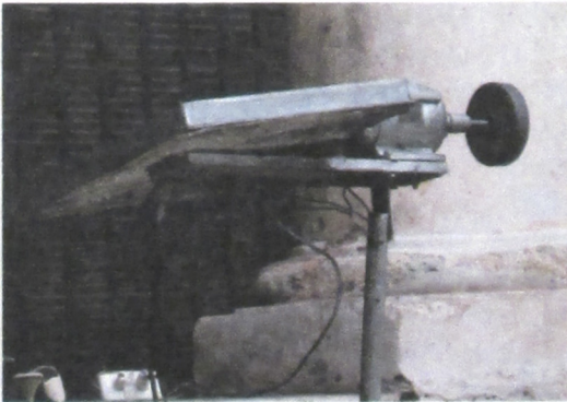
Moteurs de machines à laver Aurika utilisés comme outil par des cordonniers.
