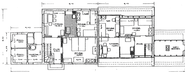
Abb. 14. Typ Alth Erd- und Obergehoß M. 1:200.
