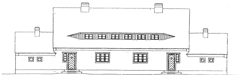
Abb. 13. Typ Alth Vorderansicht M. 1:200.
