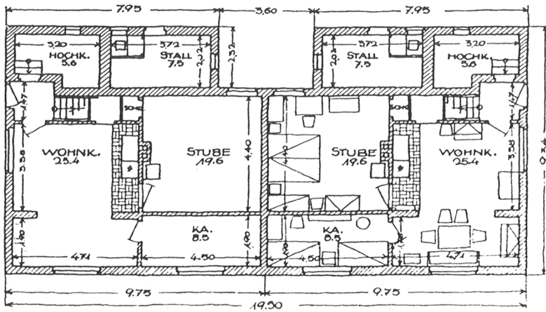
Abb. 12: Erdgeschoßgrundriß des Doppelhauses Gr. II, Form 14 L , M. 1 : 200.
